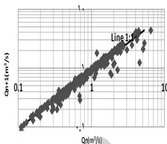
شکل ۵- نمودار فروکش بدهی جریان برای بده روز Q_n نسبت به بده روز Q_{n+1} .
