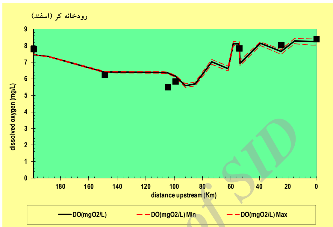
شکل ۸- اکسیژن محلول شبیه‌سازی شده در ماه اسفند
