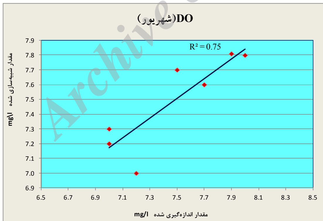
شکل ۱۱- نمودار همبستگی بین اکسیژن محلول اندازه‌گیری شده و شبیه‌سازی شده در شهریور
