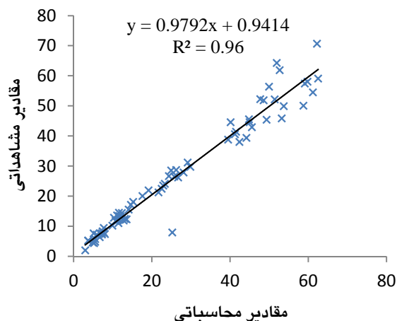
شکل ۲- مقادیر محاسباتی و مشاهده‌ای تبخیر-تعرق مرجع در مدل GP.
