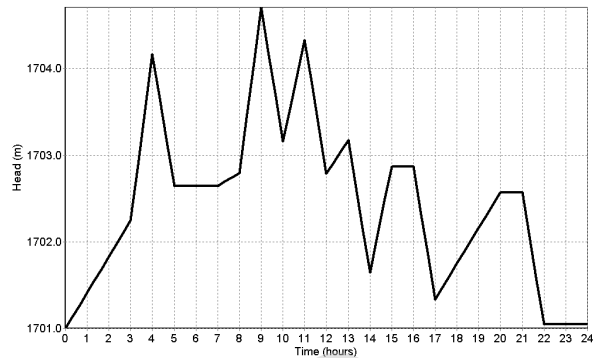
شکل ۹- تغییرات سطح آب در آبگیر ایستگاه آبکشی شماره ۳.
