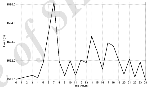
شکل ۱۰- تغییرات سطح آب در آبگیر ایستگاه آبکشی شماره ۲.
