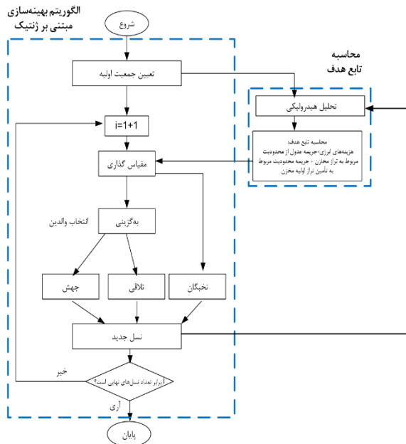
شکل ۲- روندنمای شبیه رایانه‌ای تعیین دستورالعمل نحوه بهره‌برداری بهینه از ایستگاه‌های آبکشی متوالی.
