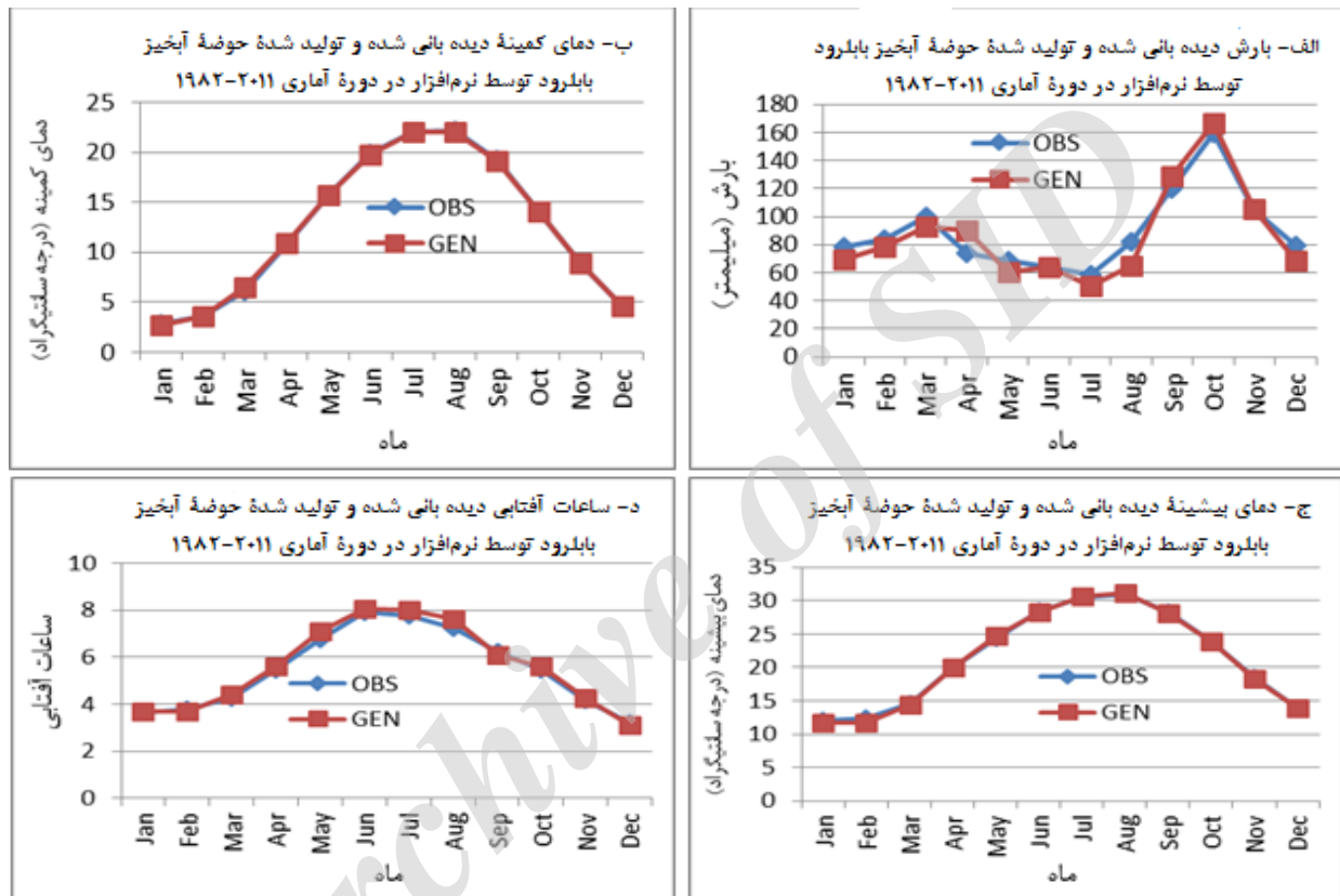
شکل ۲- مقایسه مقادیر نتایج حاصل از نرم‌افزار و دیده‌بانی شده حوضه آبخیز بابلرود جهت بررسی توانمندی نرم‌افزار LARS-WG
