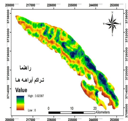
شکل ۵- نقشه‌ی تراکم آبراهه‌های محدوده مطالعه شده (کیلومتر مربع)
