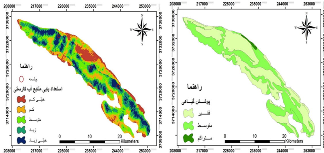
شکل ۹- نقشه‌ی استعدادیابی منابع آب کارستی محدوده‌ی مطالعه شده
