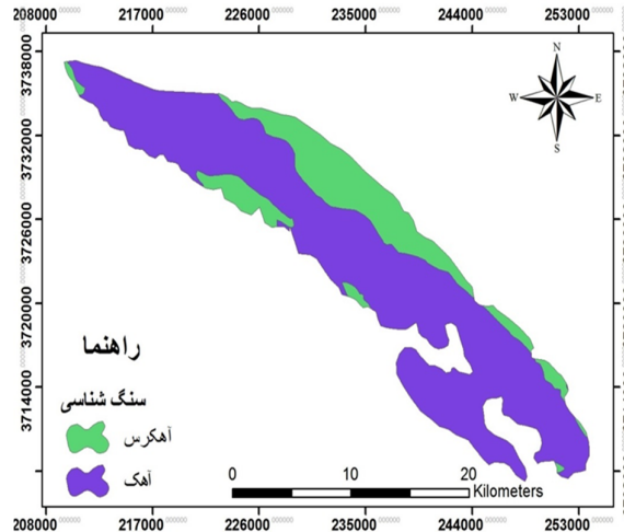
شکل ۲- نقشه‌ی سنگ‌شناسی محدوده‌ی مطالعه شده
