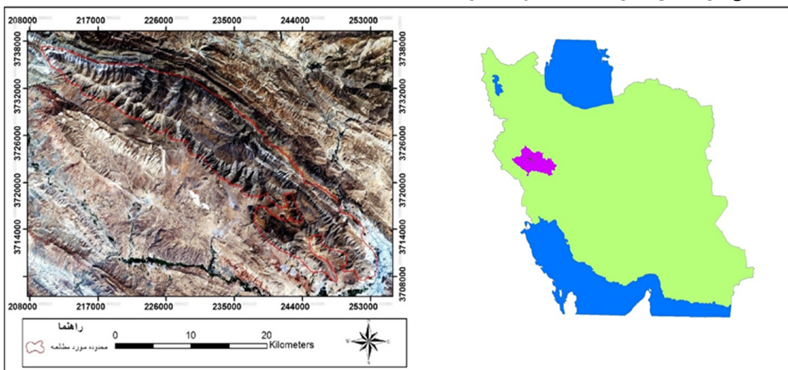
شکل ۱- موقعیت جغرافیایی تاقدیس سفیدکوه
