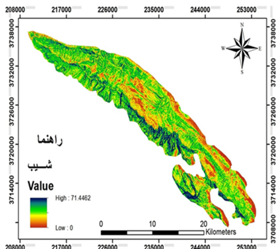
شکل ۳- نقشه‌ی درجه‌های شیب محدوده‌ی مطالعه شده
