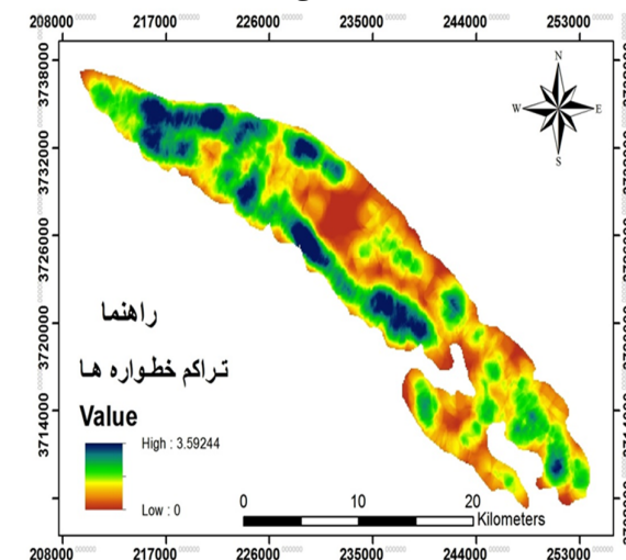
شکل ۴- نقشه‌ی تراکم خطواره‌های محدوده مطالعه شده (کیلومتر مربع)
