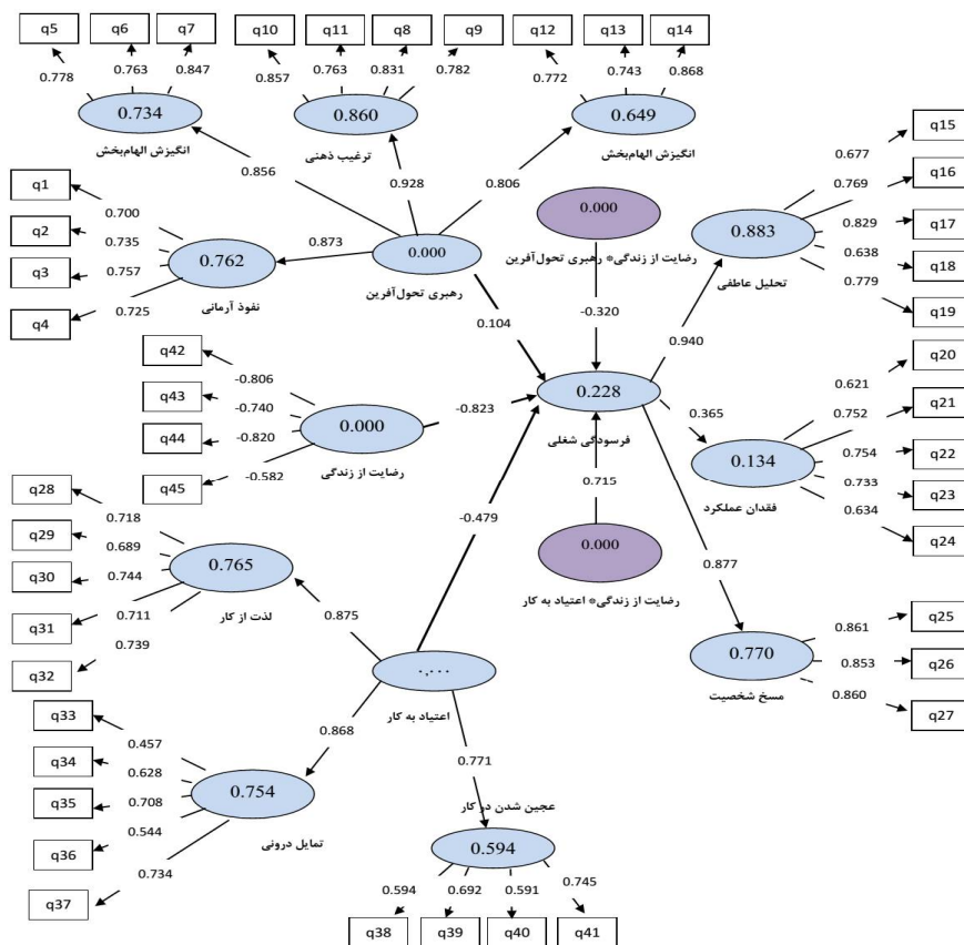
نمودار ۱- مدل در حالت تخمین ضرایب استاندارد.
