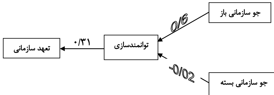
شکل ۳: ضرایب مسیر (اثرات مستقیم) مدل پرونداد
