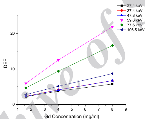
شکل ۵: فاکتور افزایش دز بر حسب غلظت‌های مختلف گادولونیوم در تمام رنج انرژی‌ها.
