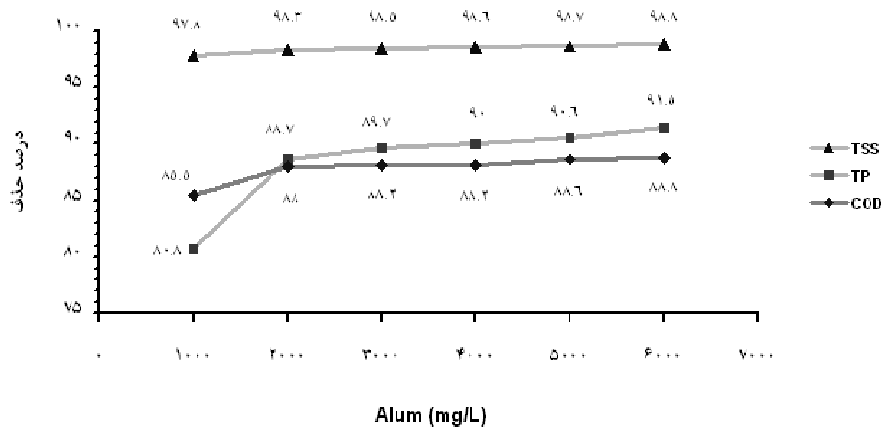
شکل ۴: نمودار تاثیر غلظت آلوم برای حذف COD, TP, و TSS در فرآیند انعقاد (pH=10)
