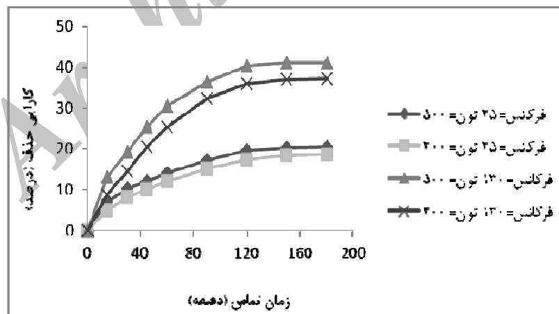
شکل ۳: تأثیر فرکانس و توان امواج اولتراسونیک بر میزان حذف بیس فنول A ( pH=11 , C_0=2mg/l )
