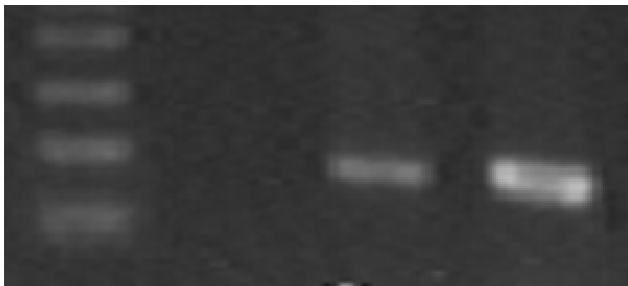
شکل ۹: تصویر ژل الکتروفورز از واکنش RT-PCR بر روی ژن DJ-1
