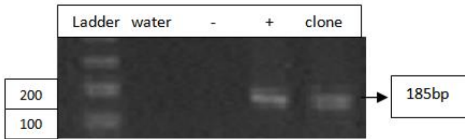
شکل ۶: واکنش PCR بر روی نمونه مثبت و نمونه مورد نظر برای ژن DJ1
