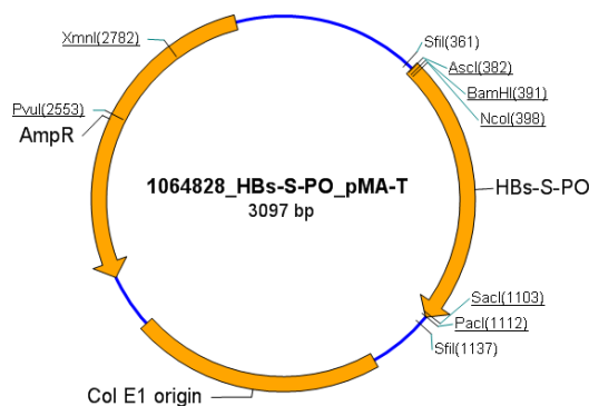
شکل ۱: توالی نوکلئوتیدی اصلاح شده آنتی ژن HBsAg برای گیاه سیبزمینی (HBs-PO) (بالا) و ناقل پلاسمیدی حاوی قطعه سنتز شده (پایین)
