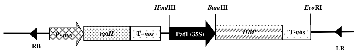
شکل ۴: نقشه سازه‌های pBI-35S-HBP و pBI-Pat-HBP. RB و LB - به ترتیب ناحیه سرحد مرزی راست و چپ، P-nos - پیشبر نوپالین سنتاز، npII - ژن مقاومت به کانامایسین، T-nos - پایانبر نوپالین سنتاز، Pat1 و 35S - به ترتیب پیشبر Patatin و CaMV35S، HBP - توالی آنتی ژن HBsAg و HindIII، BamHI و EcoRI آنزیم‌های برشی.
