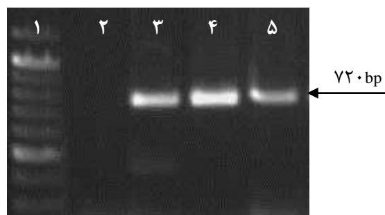
شکل ۳. تائید سازه‌های پلاسمیدی با آزمون PCR با استفاده از پرایمرهای اختصاصی HBsAg ۱- نشانگر مولکولی تعیین اندازه DNA (GeneRuler DNA Ladder, Thermo Fisher Scientific)، ۲- کنترل منفی آب، ۳- کنترل مثبت (سازه pMA-T)، ۴- pBI-35S-HBP و ۵- pBI-Pat1-HBP
