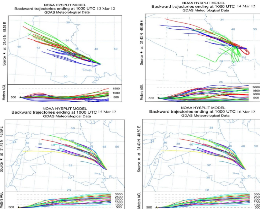
شکل شماره ۱۱: خروجی مدل HYSPLIT برای مناطق منشأ گرد و غبار ۲۳ تا ۲۶ اسفند ۱۳۹۰
