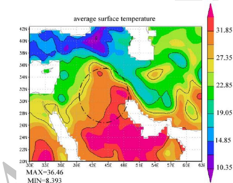
شکل شماره ۲: میانگین دمای سطح زمین در ماه اسفند (زمان وقوع توفان گرد و غبار مورخ ۱۳۹۰/۱۲/۲۳)
