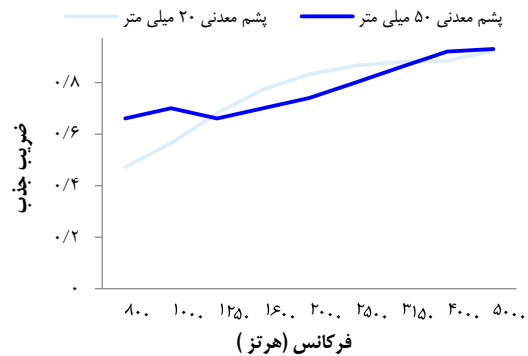
شکل ۲. ضریب جذب صوت پشم معدنی ۲۰ و ۵۰ میلی‌متر
