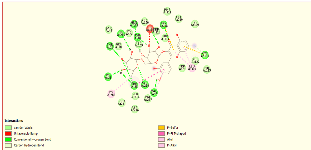
شکل ۴. برهم‌کنش‌های دوجعدی ترکیب Rutin با آنزیم آلدوز ردوکتاز (PDB ID: 1US0)
