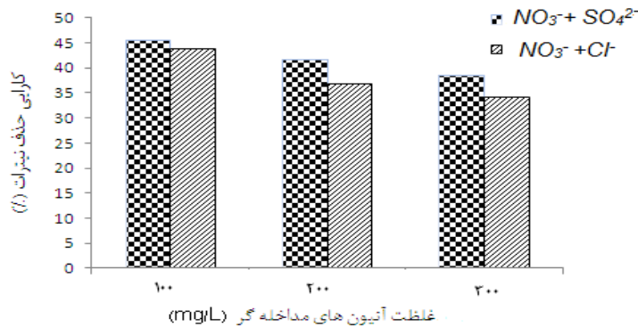
شکل ۶. اثر آبیون‌های مداخله گر در حذف نیترات (غلظت اولیه نیترات ۱۰۰، ۲۰۰، ۳۰۰ mg/l، pH=۱۰، دز ۱ g/l، زمان ۵۰ min)
