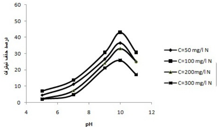
شکل ۲. تأثیر pH در واکنش (زمان ۵۰ دقیقه، مقدار پودر ۲۵/۰۰۱ گرم در لیتر غلظت‌های مختلف نیترات)
