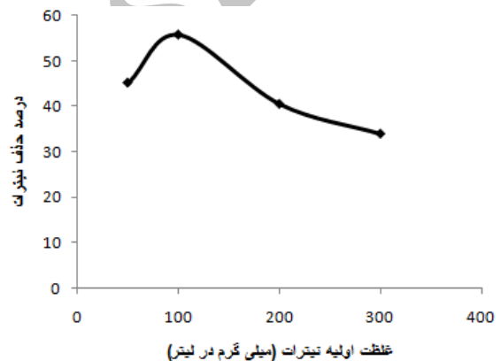
شکل ۶. تأثیر غلظت‌های مختلف نیترات ( pH=10 ، پودر آلومینیوم 1 \text{ g/l} ، زمان ۵۰ min)
