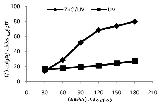
شکل ۴. مقایسه کارایی فرآیند ZnO/UV و UV تنها (ZnO=۱/۱g/l, pH=۷, C 0 =۱۰۰ mg/l)
