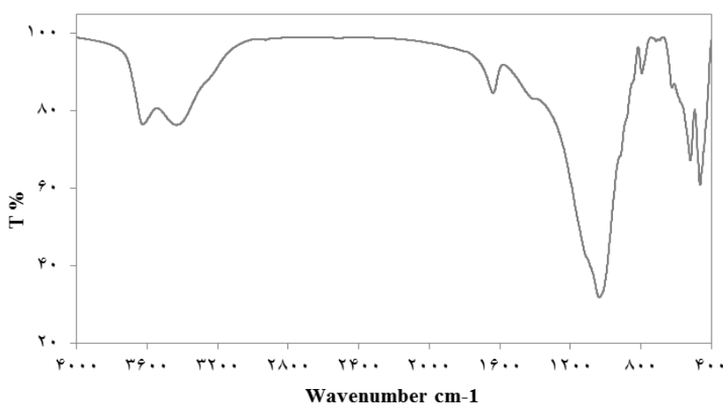
شکل ۲. طیف FTIR مربوط به جاذب GLM
