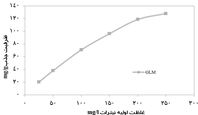
شکل ۳. اثر غلظت اولیه نیترات (دوز جذب ۱۴g/l؛ زمان تماس ۶۰ دقیقه، pH اولیه محلول ۷ و سرعت ۱۵۰ دور بر دقیقه)
