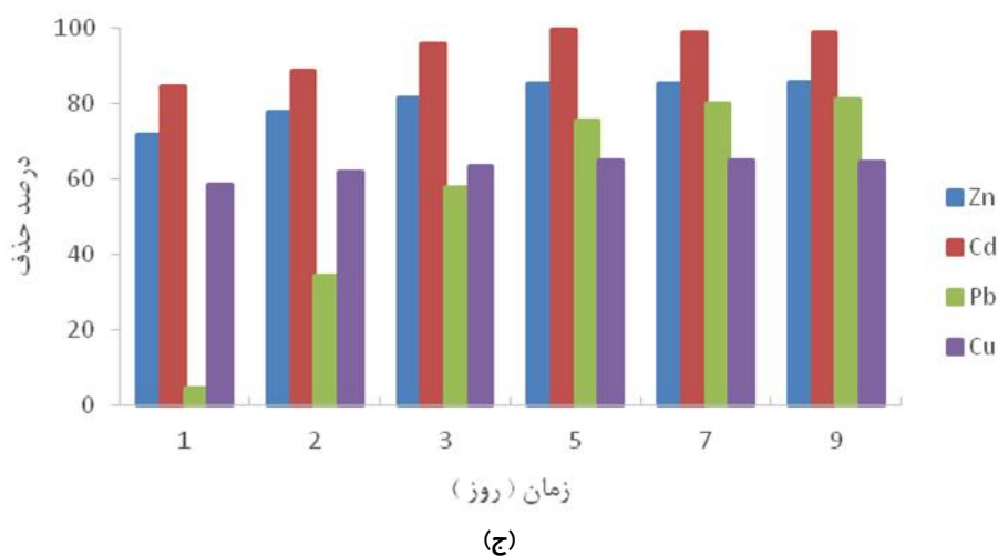
نمودار ۲. حذف فلزات سنگین از لجن فاضلاب شهری با استفاده از شستشوی بیولوژیکی در مقادیر مختلف آهن (الف=1 Fe gr/l)، (ب=2 Fe gr/l) و (ج=4 Fe gr/l) (ع)
