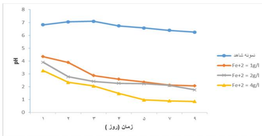
نمودار ۱. تغییرات pH با تغییر غلظت آهن در حین فرایند شستشوی بیولوژیکی با اسید تیوباسیلوس فرواکسیدانت
