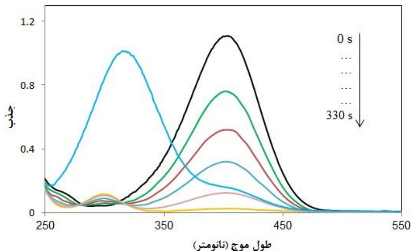
شکل ۷. طیف UV-Vis از محلول آبی \text{E} - نیترو فنول در حضور ۲۵۰ میلی مولار \text{NaBH}_4 و ۱۰/۰ میلی گرم نانو کامپوزیت نقره- اکسید روی بیوسنتز شده (منحنی های رنگی در طول موج ۴۰۰ نانومتر، کاهش پیک جذبی مربوط به \text{E} - نیترو فنول را در طی واکنش حذف نشان می دهند).
