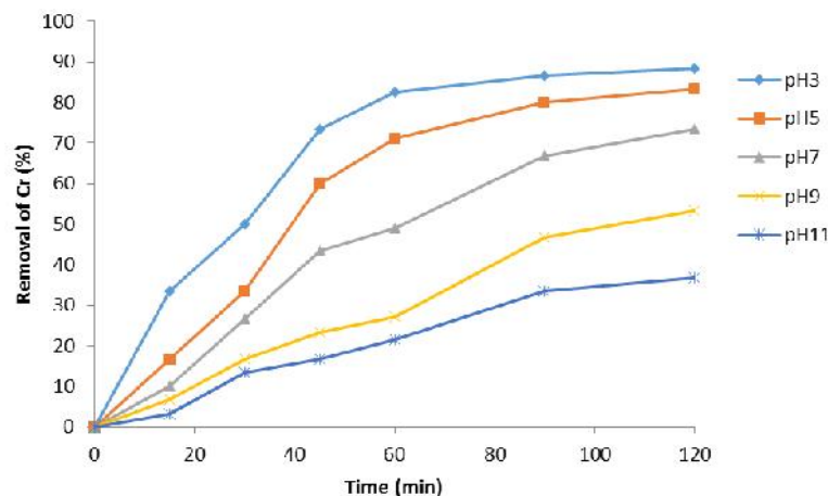
نمودار ۱. تأثیر pH بروی فرایند حذف فتوکاتالیستی کروم شش ظرفیتی (غلظت اولیه کروم شش ظرفیتی ۳۰ mg/l و مقدار اولیه نانوکامپوزیت ۱ g/l)
