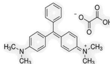
شکل ۱. ساختار مولکولی مالاشیت سبز
