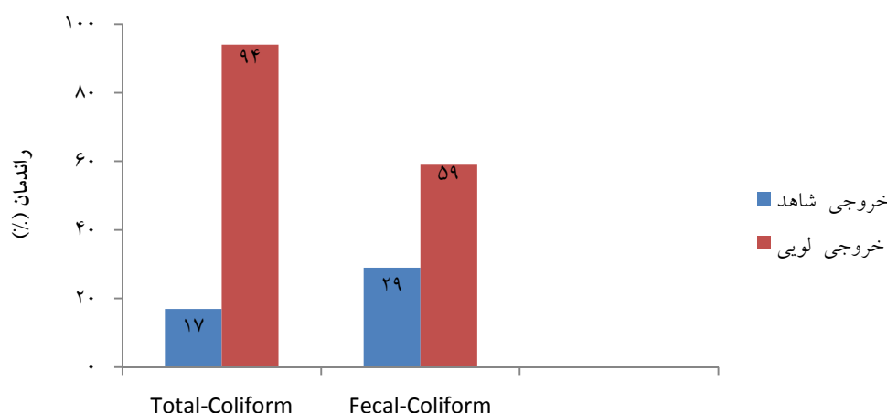
نمودار ۳: راندمان حذف کلیفرم کل و کلیفرم گوارشی
