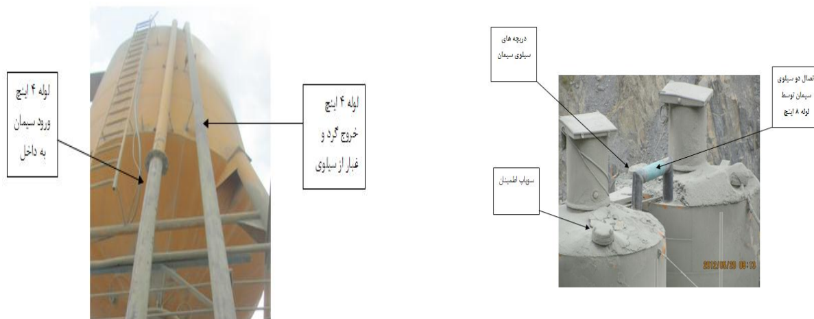
شکل ۳: اتصال دو سیلوی سیمان توسط لوله ۸ اینچ
