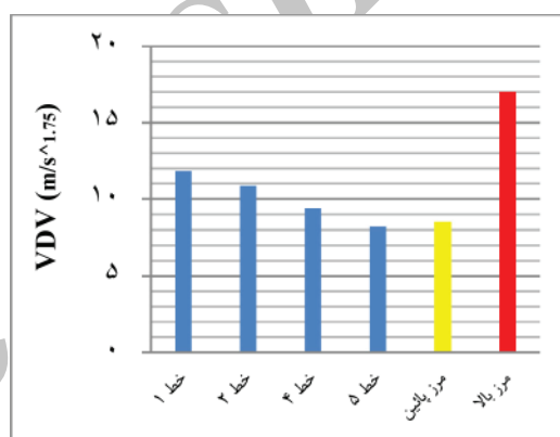
شکل ۳: مقایسه میانگین مقادیر VDV در خطوط مختلف مترو با حدود بالا و پایین HGZ
