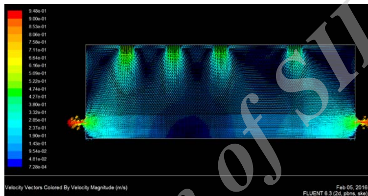
شکل ۴. نتایج شبیه سازی الگوی جریان هوا در اتاق پاک راهرو (کلاس D)
