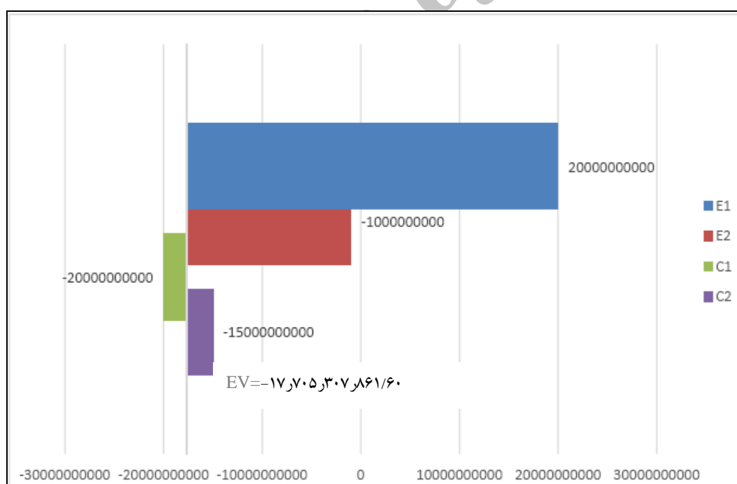
نمودار ۱: تورنادو
