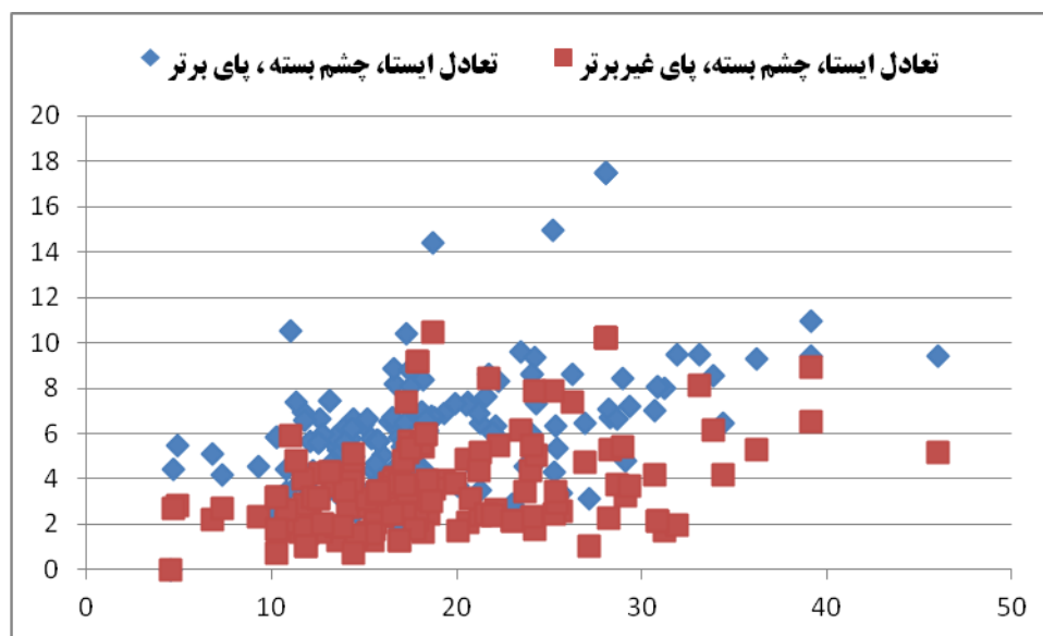
نمودار ۳. پراکندگی نقطه‌ای تعادل ایستا با چشم بسته در ۲ موقعیت پای برتر و غیر برتر
