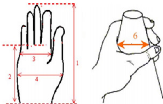
شکل ۱. ابعاد آنتروپومتریکی اندازه‌گیری شده در مطالعه حاضر (۱. طول دست، ۲. طول کف دست، ۳. عرض کف دست، ۴. عرض دست، ۵. طول انگشتان و ۶. قطر چنگش)
