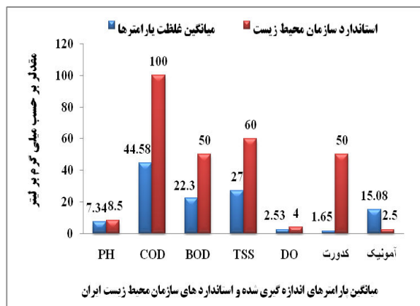
نمودار ۸: نمودار مقایسه میانگین پارامترهای اندازه گیری شده با استاندارد های سازمان محیط زیست ایران
