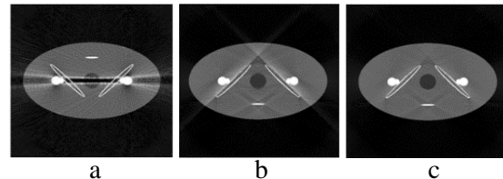
شکل ۶: اصلاح آرتیفکت فلز در فانتوم لگن در پژوهش Peng a: تصویر فانتوم لگن همراه با فلز و بدون اصلاح b: تصویر اصلاح شده به روش L1. c: تصویر اصلاح شده به روش NMAR
