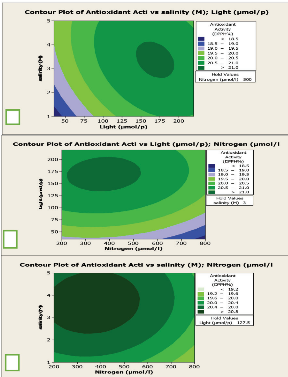
شکل شماره ۱- اثرات متقابل: (a) شوری × شدت نور بر میزان آنتی اکسیدان موجود در جلبک دونالیلا سالینا در میزان نیتروژن ثابت ۵۰۰ میکرومول بر لیتر، (b) شوری × میزان نیتروژن بر میزان آنتی اکسیدان موجود در جلبک دونالیلا سالینا در میزان شدت نور ثابت ۱۲۷/۵ میکرومول فوتون و (c) شدت نور × میزان نیتروژن بر میزان آنتی اکسیدان موجود در جلبک دونالیلا سالینا با میزان شوری ثابت ۳ مولار.
