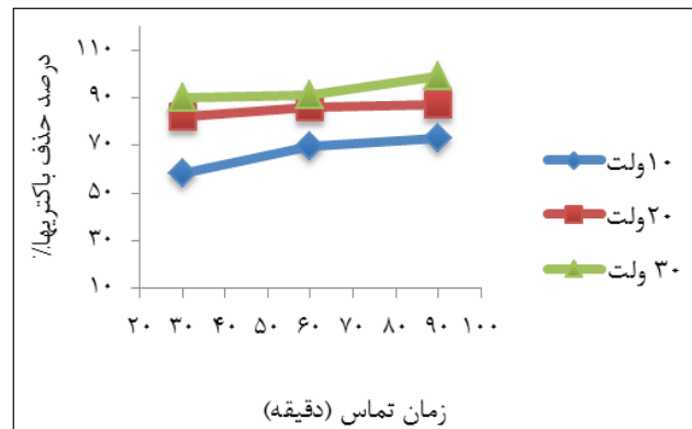
نمودار ۱: درصد حذف باکتری‌ها با تغییرات زمان ماند
