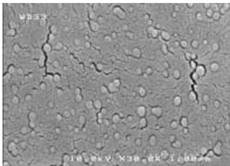
شکل ۲: توزیع نانوذرات چیتوزان حامل پاکلی تاکسل در محیط خشک که با میکروسکوپ الکترونی اندازه‌گیری شده است.
