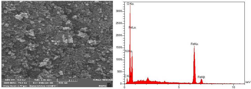
شکل ۱: عکس SEM-EDS نانو ذرات مگنتیک سنتز شده
