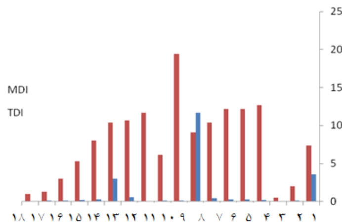
نمودار ۱: نمودار غلظت در کارگاههای مختلف بر حسب mg/m 3
