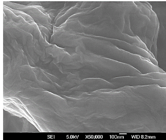
شکل ۱: تصویر SEM گرافن اکساید (GO)
