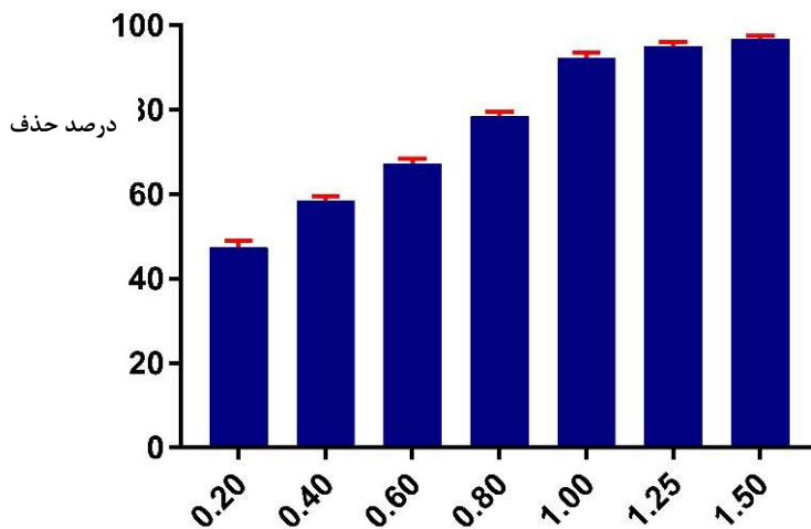
نمودار ۴: تأثیر زمان تماس روی جذب (pH=۶، غلظت ۵۰ میلی گرم بر لیتر، دز جاذب ۰/۲ گرم بر لیتر)
