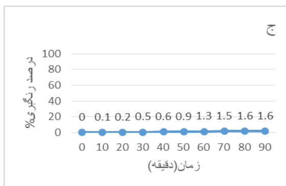
نمودار ا: الف) اثر میزان رنگبری در حضور نور UV به تنهایی ب) اثر فتوکاتالیست به تنهایی ج) اثر هیدروژن پر اکسید بدون حضور نور UV
