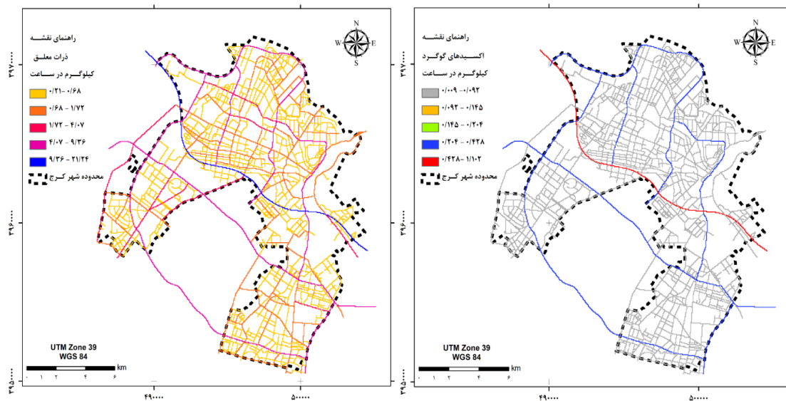
شکل ۷: توزیع انتشار اکسیدهای گوگرد و ذرات معلق ناشی از وسایل نقلیه در حال تردد در شهر کرج در ساعات اوج ترافیک صبح در شبکه‌های ۵۰ متر در ۵۰ متر
