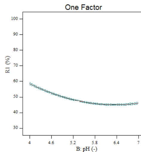
شکل ۴: تأثیر pH بر راندمان حذف ایبوپروفن
