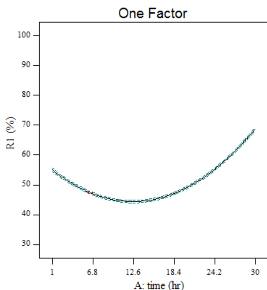
شکل ۵: تأثیر زمان بر کارایی حذف ایبوپروفن
