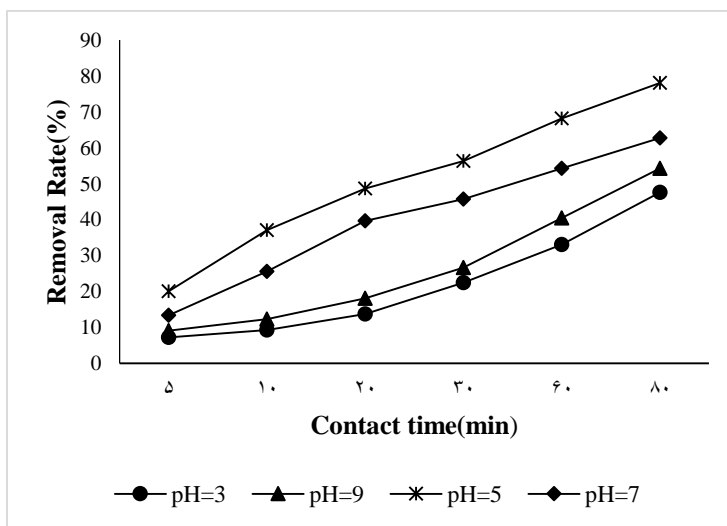
شکل ۳: نتایج مربوط به تاثیر pH اولیه بر کارایی حذف جیوه با استفاده از MBSA (غلظت اولیه جیوه ۵۰۰ میکروگرم بر لیتر، دوز جاذب ۰/۱ گرم بر لیتر، دمای ۲۵ درجه سلسیوس)
