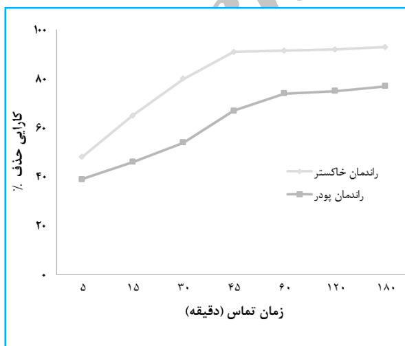
نمودار ۳. تأثیر زمان تماس بر روی میزان کارایی حذف رنگ راکتیو آبی ۲۹ (pH=۳، دوز جذب ۴ g/L، غلظت رنگ ۲۵ mg/L)
