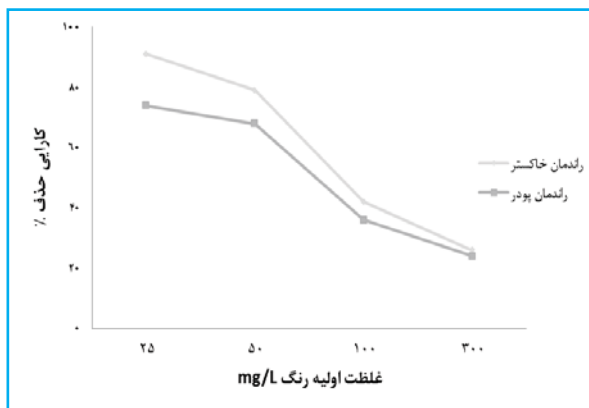
نمودار ۲. تأثیر تغییرات غلظت اولیه رنگ راکتیو آبی ۲۹ بر روی میزان کارایی حذف (pH=۳، زمان تماس برای پودر ۶۰ min و برای خاکستر ۴۵ min)
