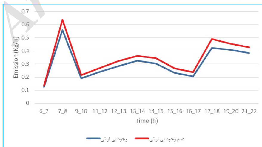
شکل ۱۲. مقایسه میزان انتشار بنزن در دو سناریو
