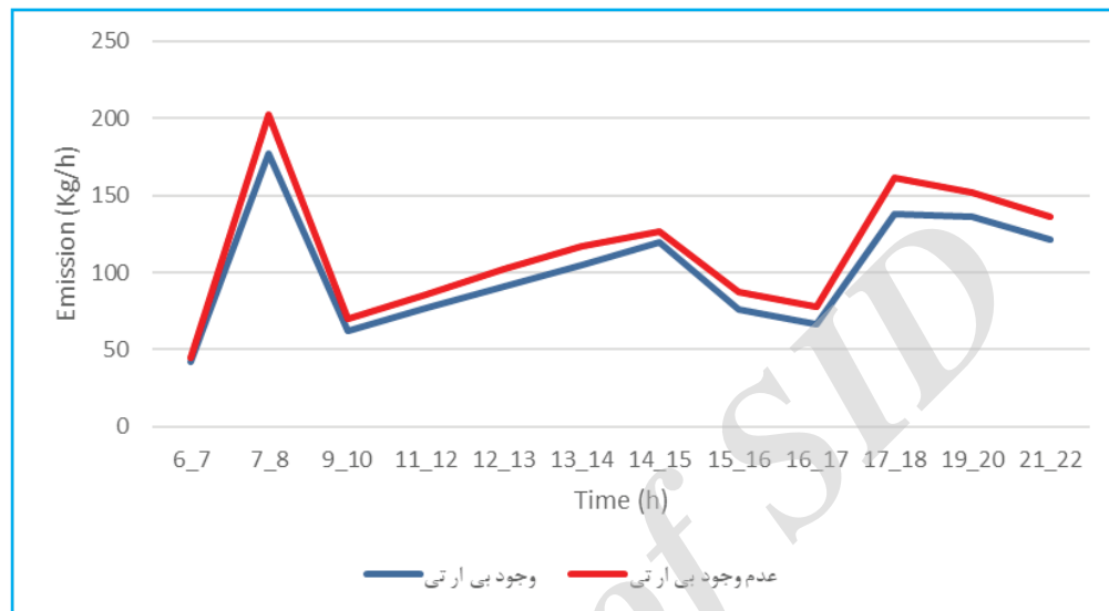
شکل ۷. مقایسه میزان انتشار مونوکسیدکربن در دو سناریو
