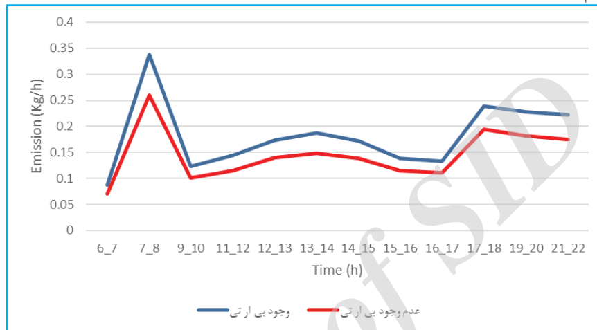
شکل ۱۱. مقایسه میزان انتشار ذرات کمتر از ۱۰ \mu در دو سناریو
