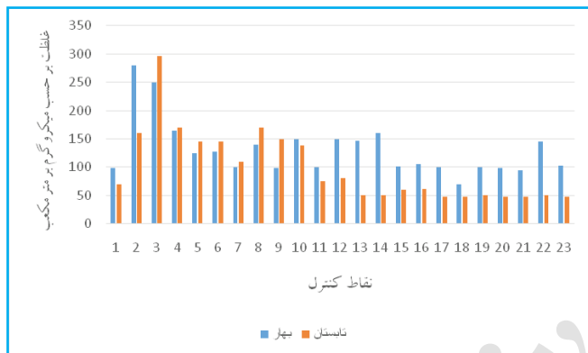
نمودار ۳. تغییرات فصلی مقادیر غلظت محیطی PM 10
