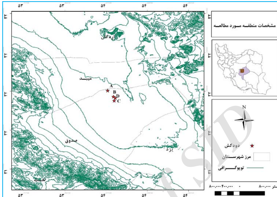
شکل ۱. مشخصات منطقه مورد مطالعه و توپوگرافی منطقه
