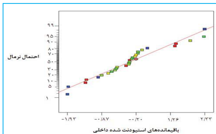
نمودار ۱ الف). ارتباط بین درصد مقادیر تجربی و پیش‌بینی شده (توسط RSM) حذف ۶،۴،۲-تری‌کلوروفنول توسط فرآیند فوتوکاتالیستی
