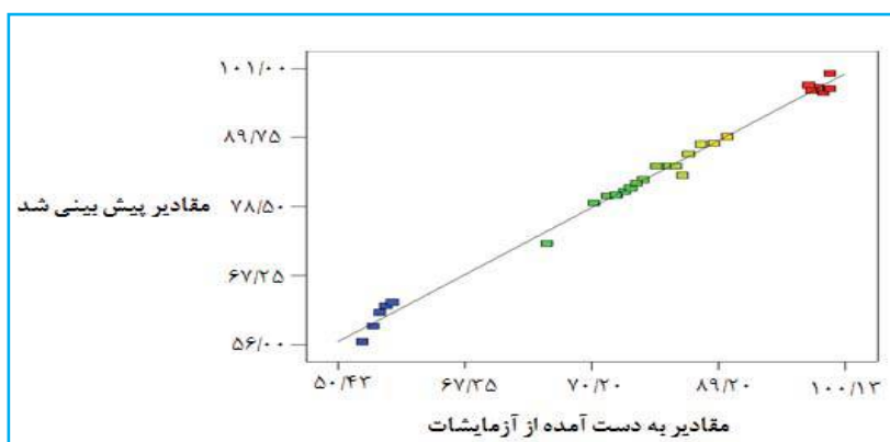
نمودار ۱ ب). نمودار توزیع احتمال نرمال برای باقی‌مانده‌های حذف ۶،۴،۲-تری‌کلوروفنول توسط فرآیند فوتوکاتالیستی
