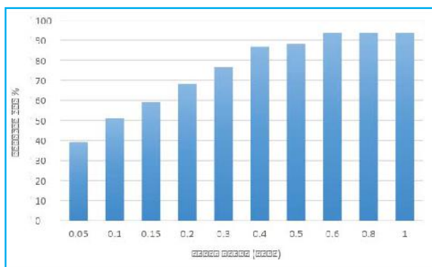
نمودار ۲. راندمان حذف پنی سیلین G در جریان الکتریکی مختلف در فرآیند الکترو-فنتون (غلظت ۱۰۰ میلی گرم بر لیتر، pH=۳، فاصله بین الکتروها ۱ سانتی متر و ولتاژ ۲۶ ولت در ۱۵ دقیقه)
