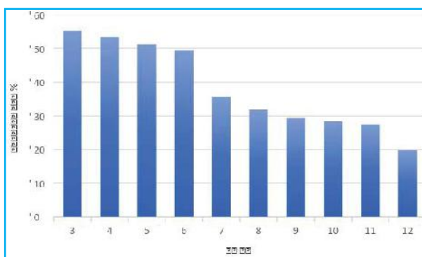
نمودار ۱. راندمان حذف پنی سیلین G در pHهای مختلف در فرآیند الکترو-فنتون
