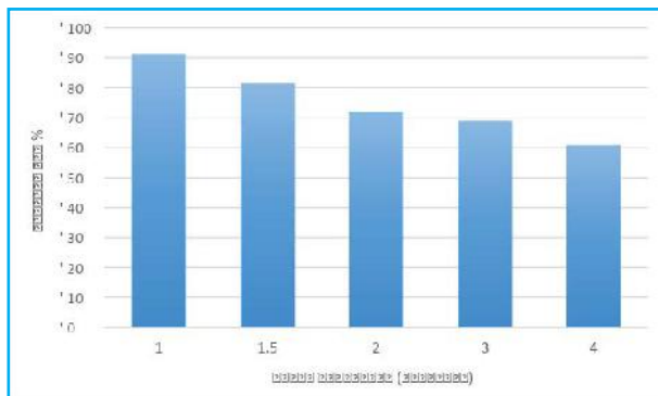
نمودار ۵. راندمان حذف پنی سیلین G در فاصله الکترودها اولیه مختلف در فرآیند الکترو-فنتون (غلظت ۵۰ میلی گرم بر لیتر، جریان ورودی ۰/۶ آمپر، pH=۳، ولتاژ ۲۶ ولت در ۲۰ دقیقه)
