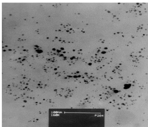
شکل ۵- شکل و اندازه نانوذرات نقره تولید شده با عصاره آبی گل اکالیپتوس کامالدولنسیس توسط میکروسکوپ الکترونی نگاره
