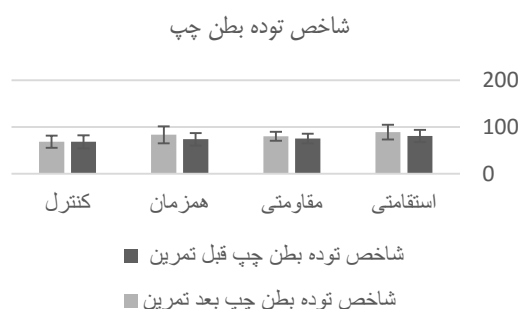
نمودار ۲. مقایسه میانگینهای شاخص توده بطن چپ، قبل و بعد از اجرای برنامه های تمرینی
