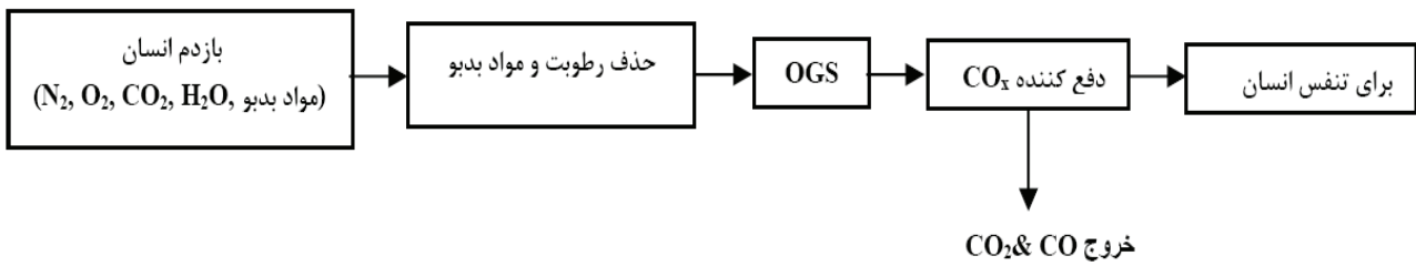
شکل ۱. نمایی از نمودار جریان تولید اکسیژن از بازدم انسان
