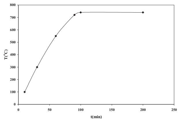
شکل ۳. پروفیل دمایی OGS در جریان ۱۴۰ mA
