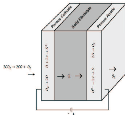
شکل ۲. اساس عملکرد الکترولیزور اکسیدی جامد [۱۵]
